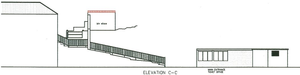
ELEVATION C-C
